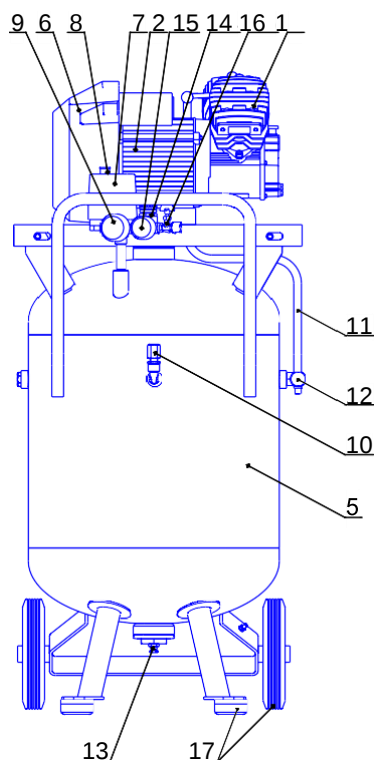
Рисунок 11 - Общий вид компрессора СБ4/С-100.J2047BB
