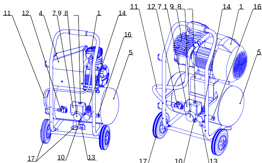
Рисунок 11 - Общий вид компрессора СБ4/С-100.J2047BB
