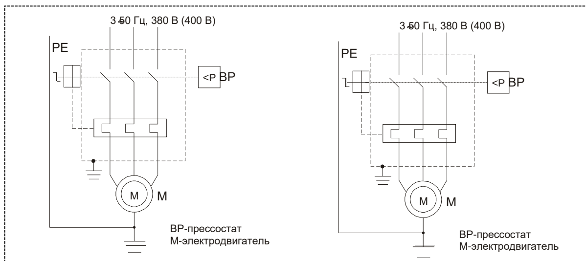
Рисунок А.2 – Схема электрическая принципиальная компрессора СБ4/Ф-500.LB75TB
